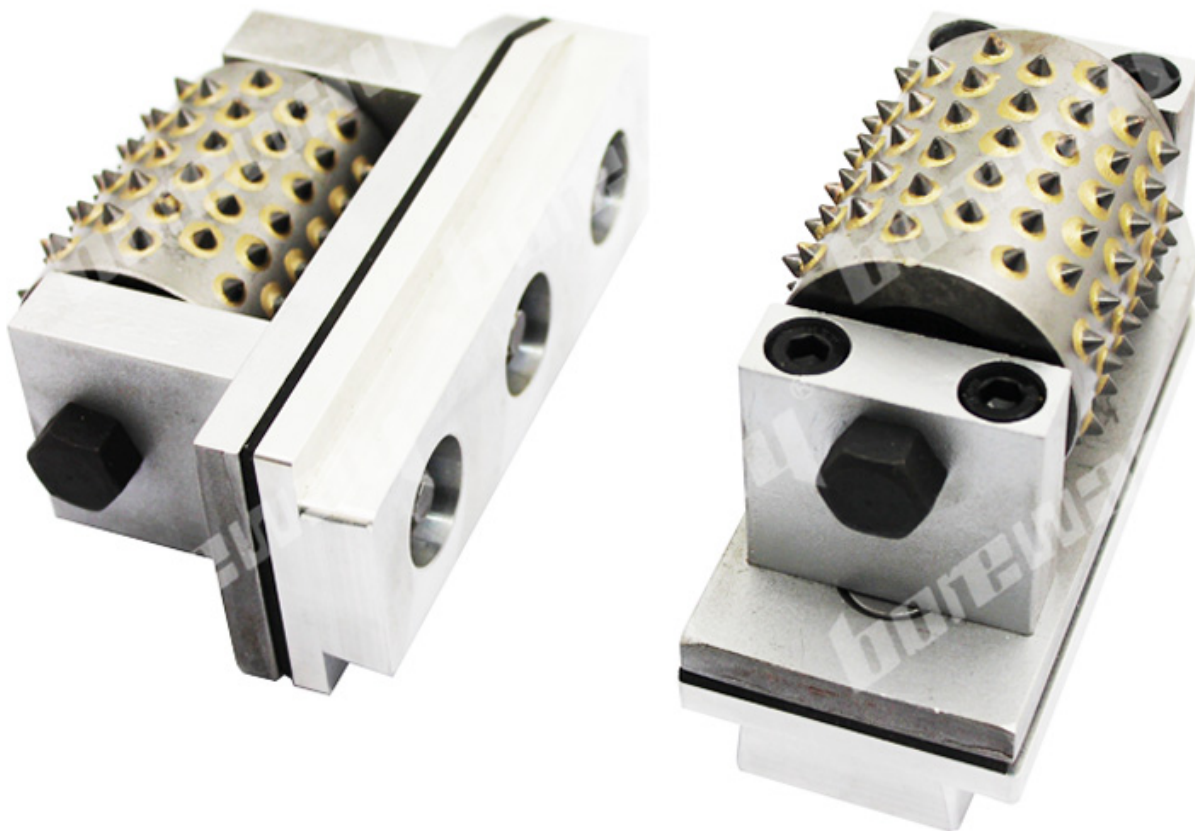
Cabezal de rodillo de molienda con 99 segmento para moler y calibrar las losas de piedra como granito, mármol, etc.
