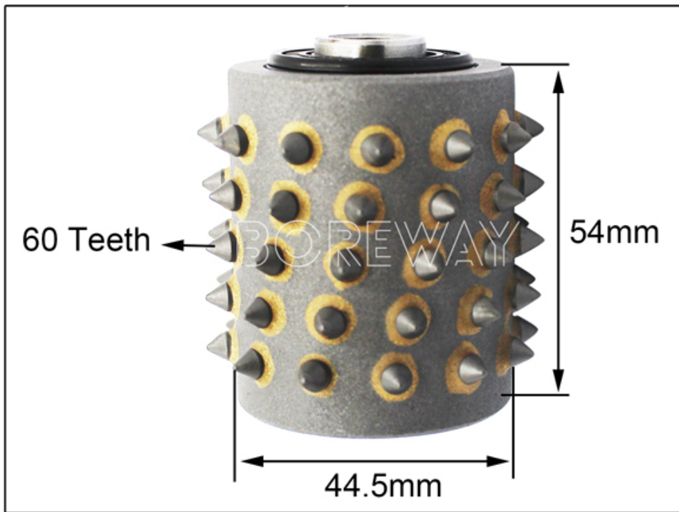
60 Teeth
