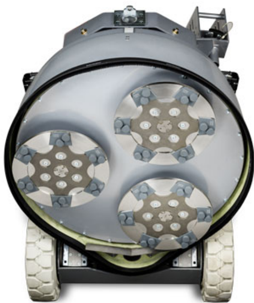
Utensile diamantato Lavina con segmenti PCD a doppio quarto e segmento a una barra
